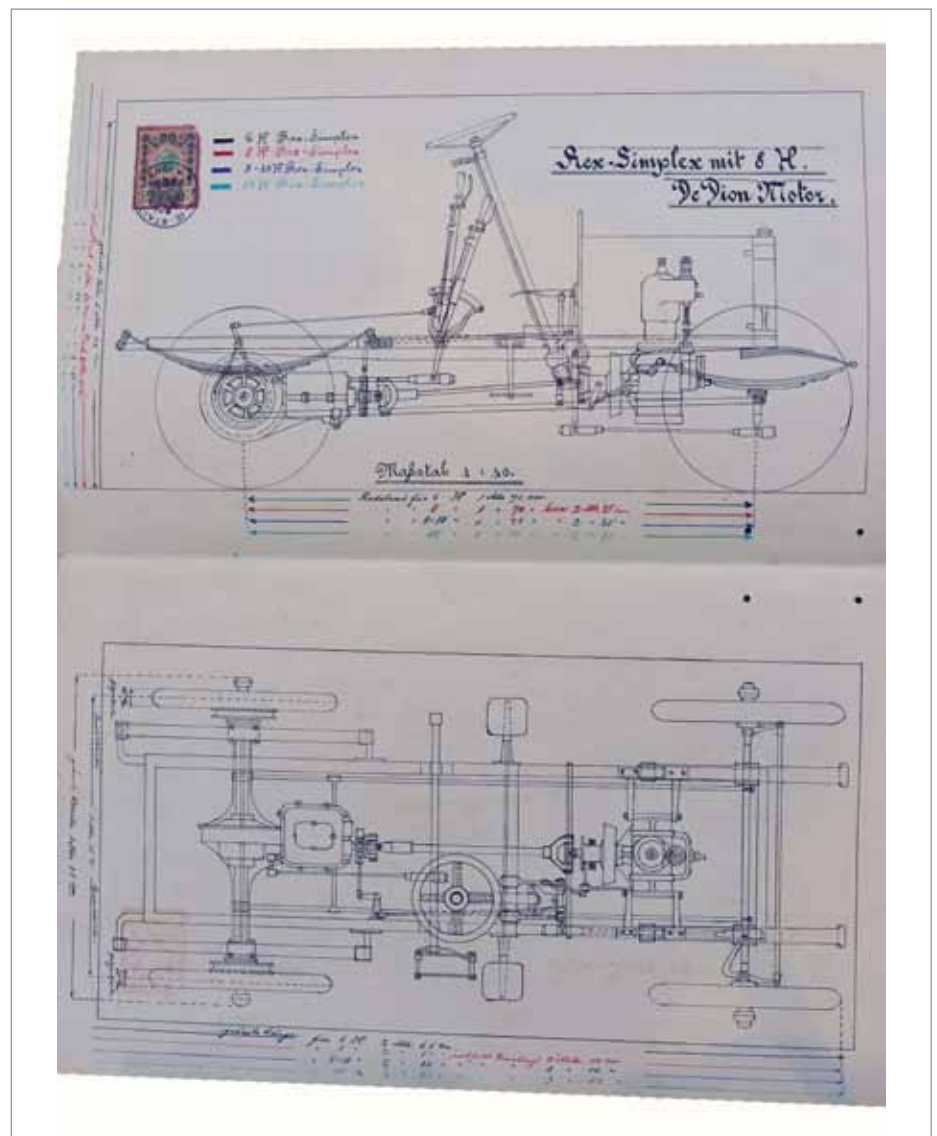
(NÖLA, NÖ Reg XIII 1447/1905-X-146; Karton 1339) „Typenschein“ - maßstabsgetreuer Tuschezeichnung eines Rex Simplex.
